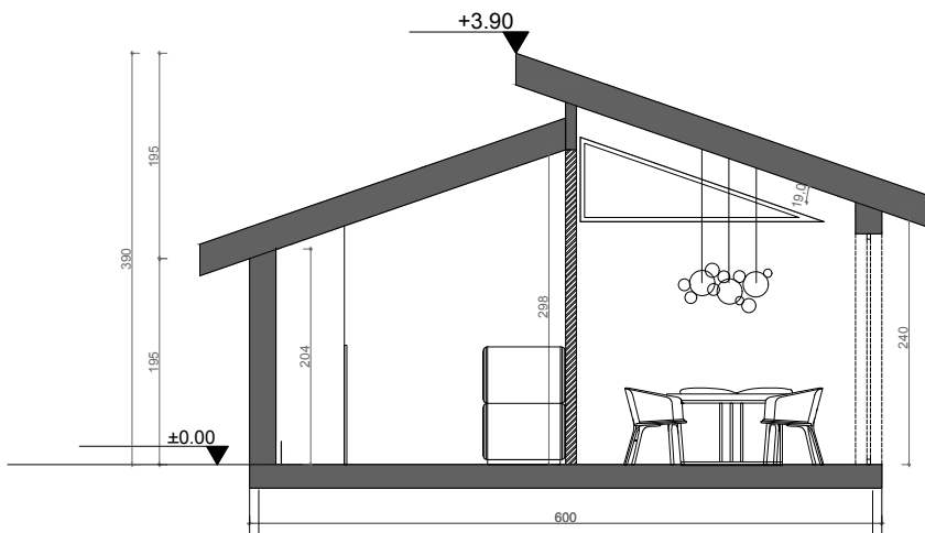
PRZEKRÓJ A-A
