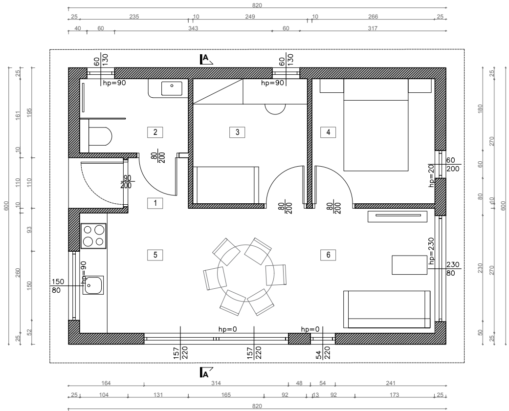
RZUT PARTERU
