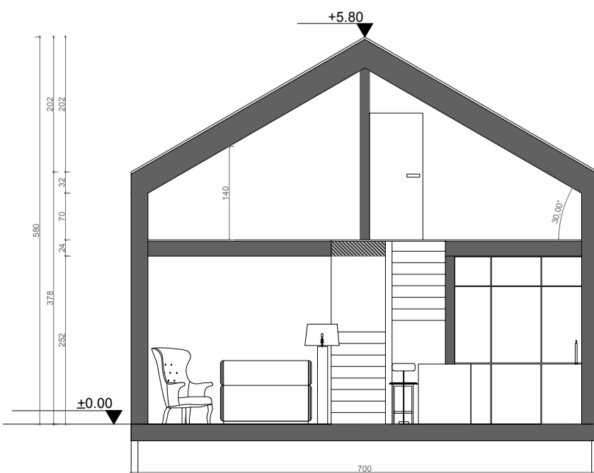
PRZEKRÓJ A-A
