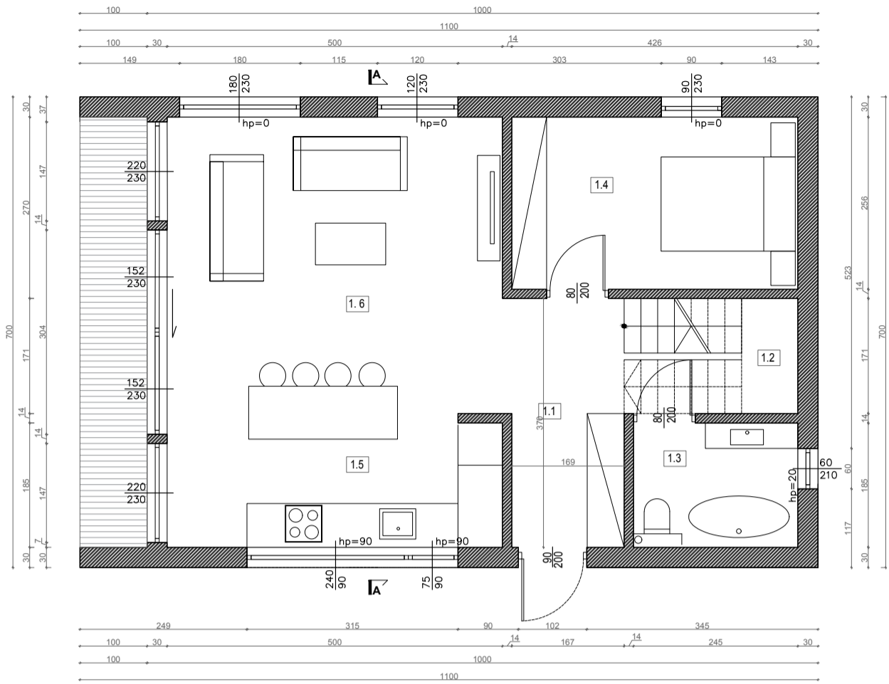
RZUT PARTERU
