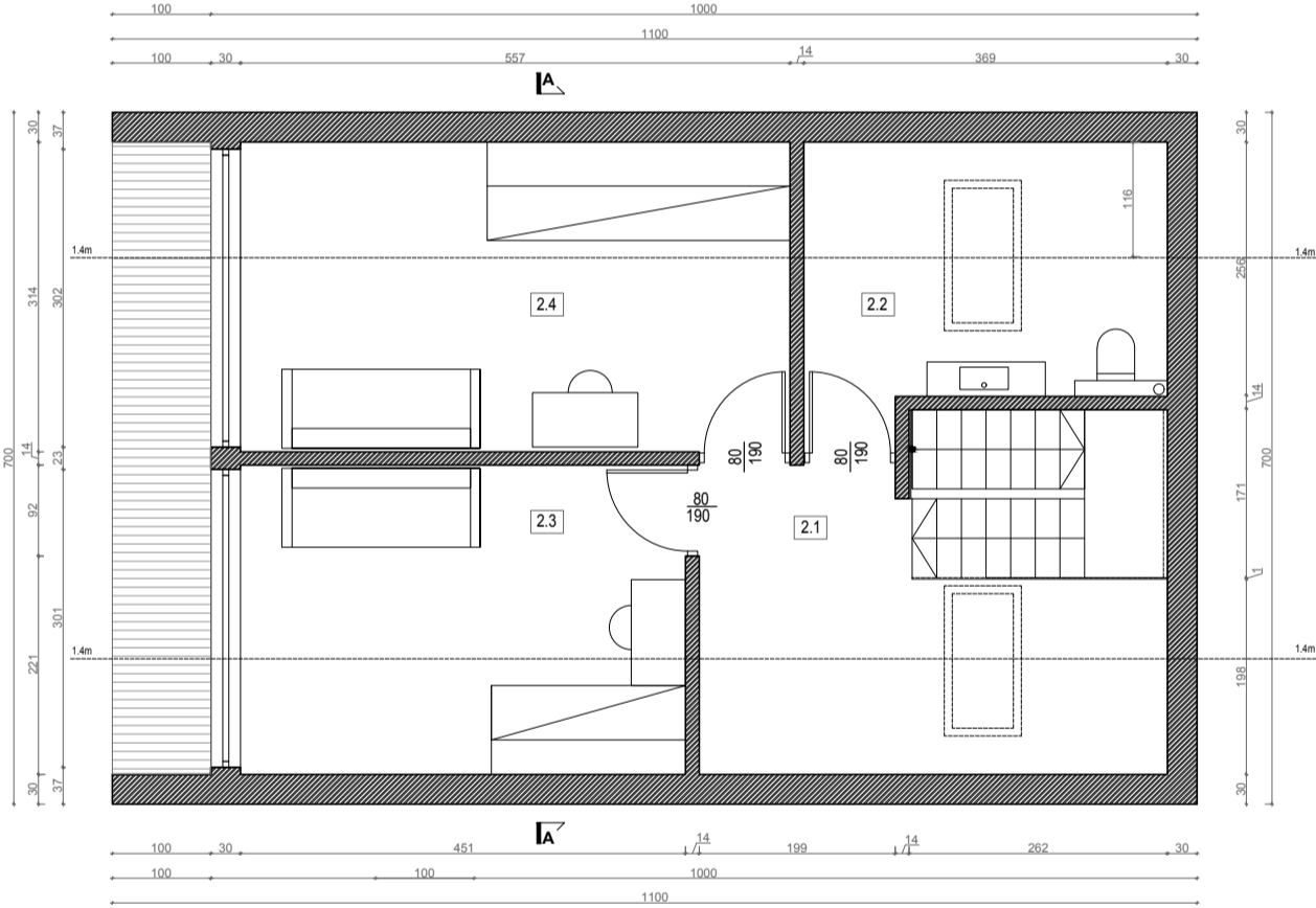
RZUT ANTRESOLI
