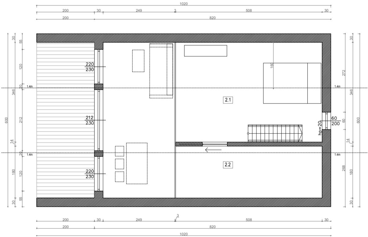
RZUT ANTRESOLI
