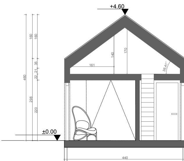
PRZEKRÓJ A-A
