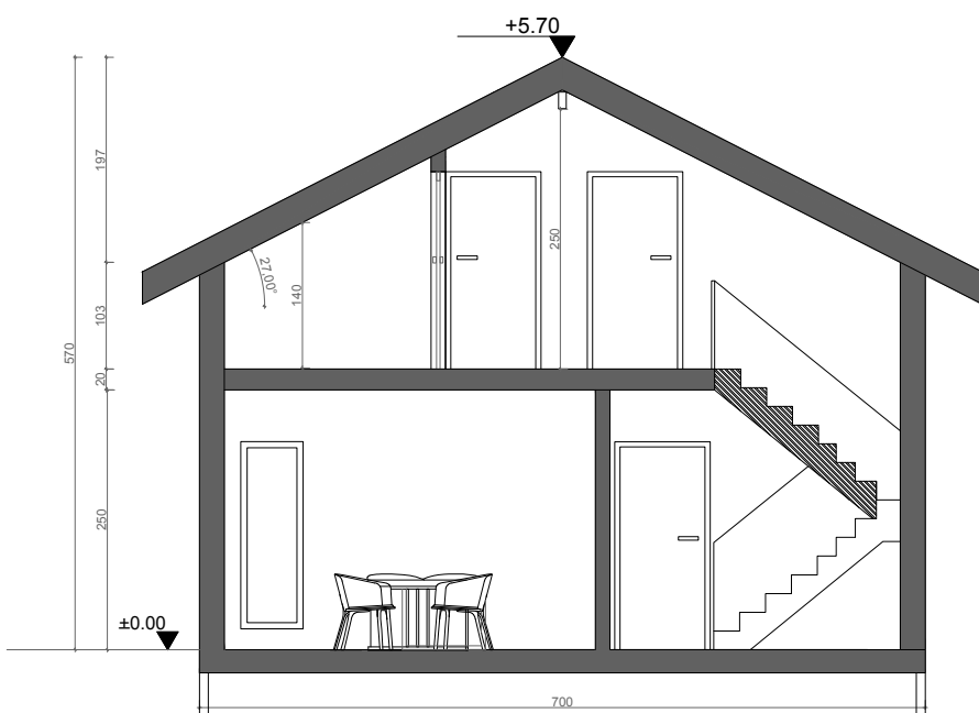
PRZEKRÓJ A-A
