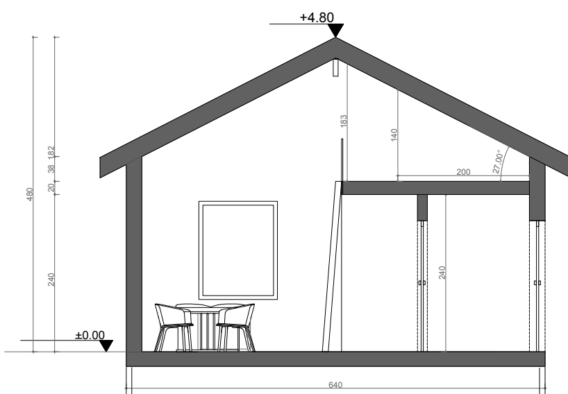
PRZEKRÓJ A-A
